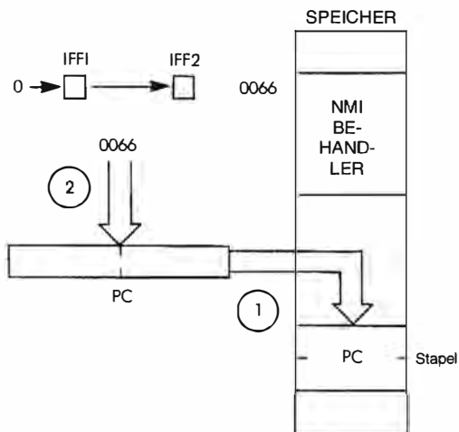
Abb. 6.25: Der NMI erzwingt eine automatische Verzweigung
