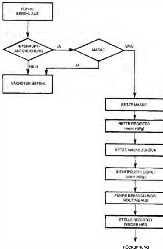
Abb. 6.34: Interruptlogik
