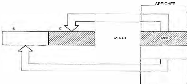
Abb. 3.15: LD BC, (MPRAD)
