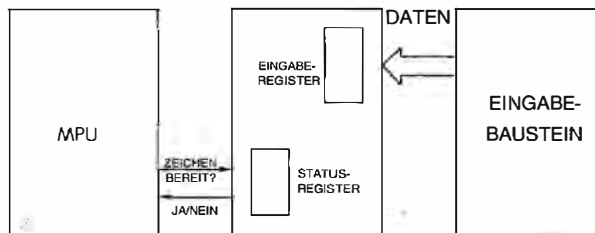
Abb. 6.8a: Handshaking (Eingabe)
