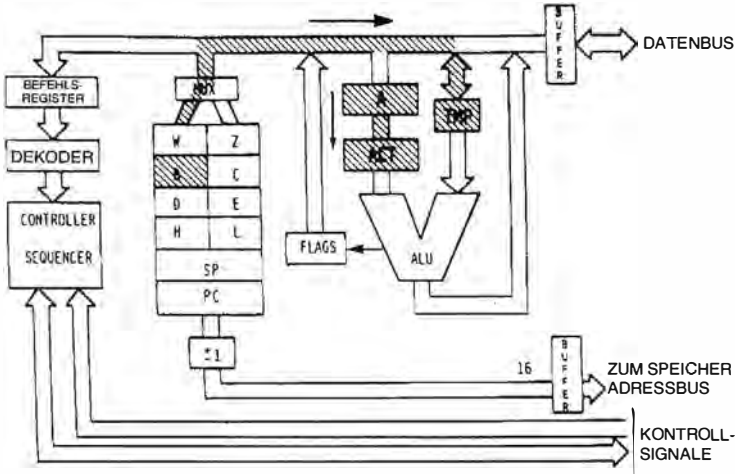
Abb. 2.23: Zwei Transfers werden gleichzeitig ausgeführt
