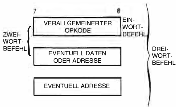
Abb. 2.15: Typisches Befehlsformat
